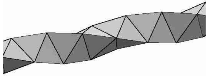
Fig. 8. The Boerdijk-Coxeter helix.
